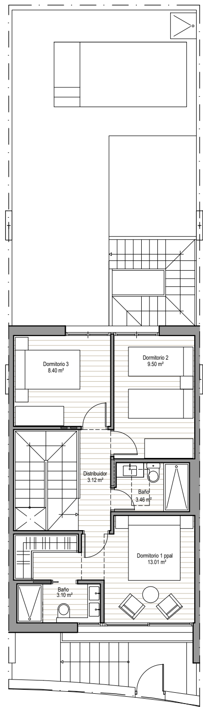
PLANTA ALTA
