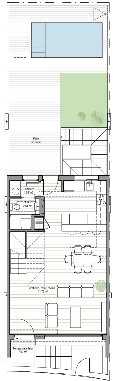
PLANTA BAJA
